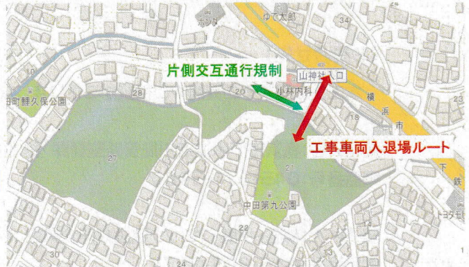
図②: 計画変更後発進立坑工事ヤード
